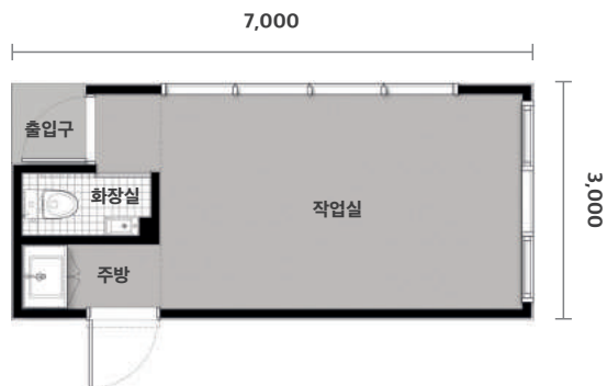
평면도 | 좌측형
