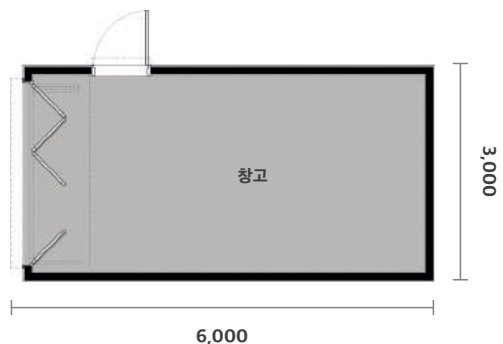
평면도 | 좌측형
